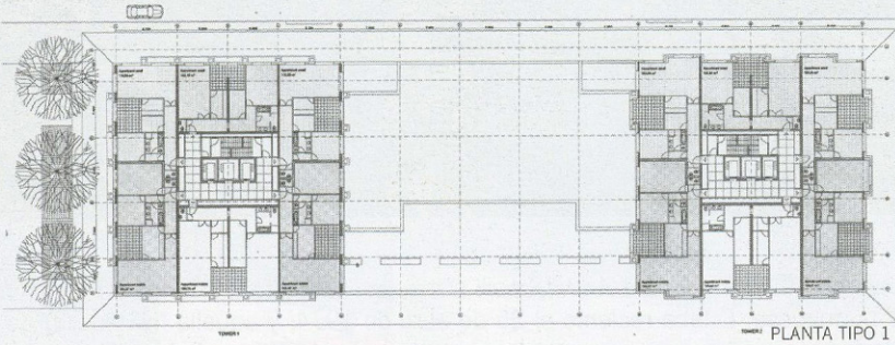
PLANTA TIPO 1
