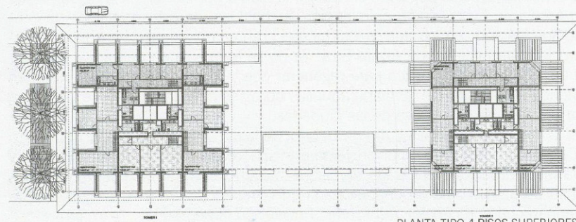
PLANTA TIPO 4 PISOS SUPERIORES
