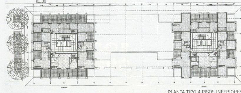
PLANTA TIPO 4 PISOS INFERIORES
