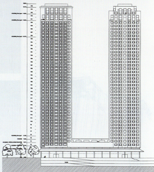
35 · ALZADO FRONTAL
