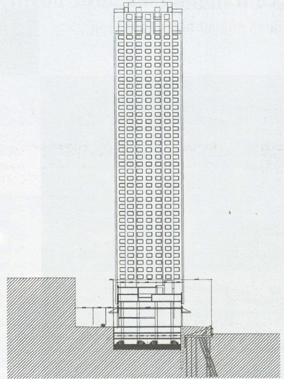
37 · SECCION TORRE 2
